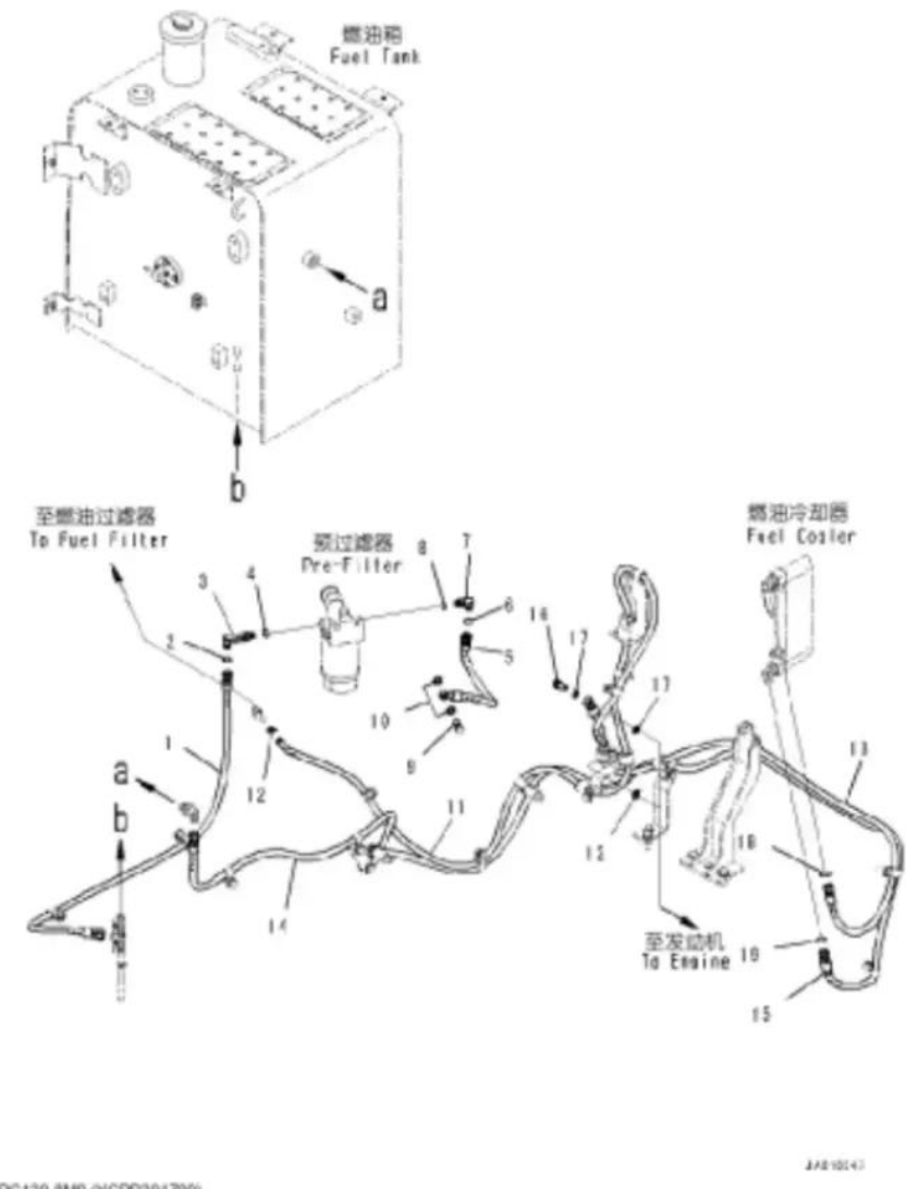
图号 D0200-001001 供油管路 (燃油管路) FIG. D0200-001001 Fuel Supply Piping (Fuel Piping)
