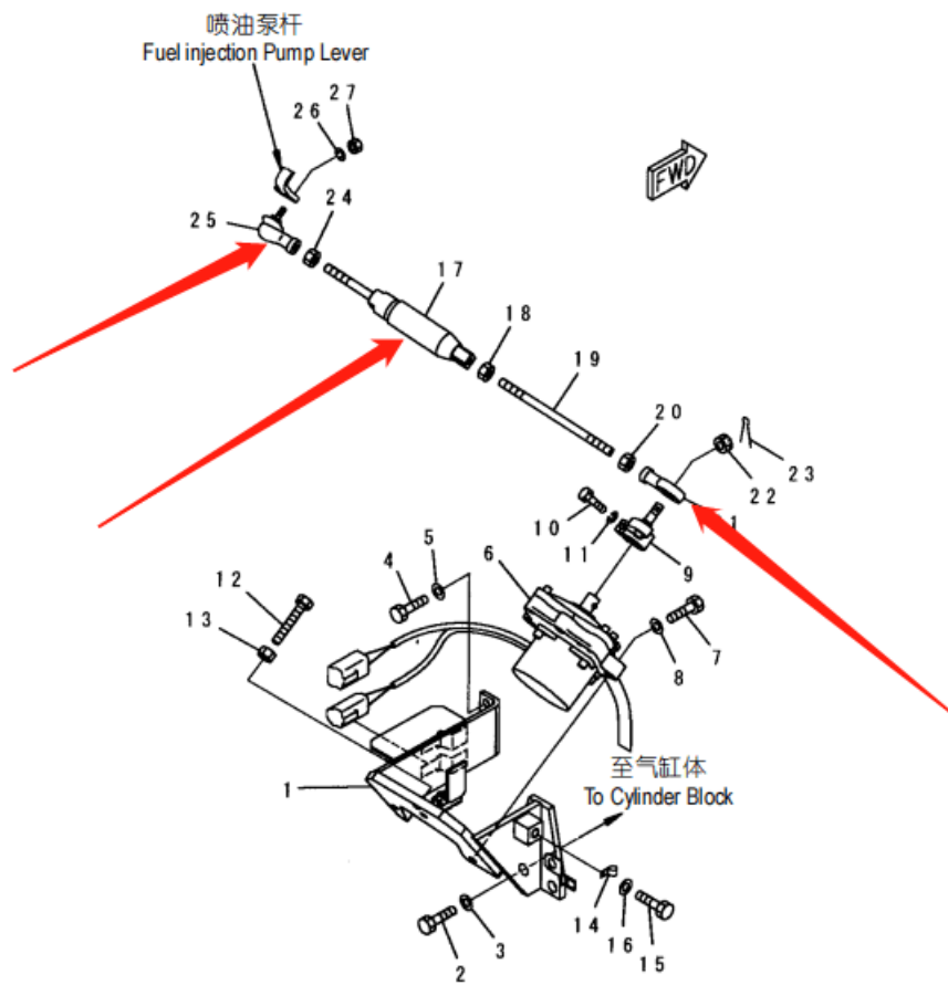
FIG. BO400-01A0 燃油控制装置 FUEL CONTROL
