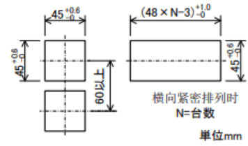
面板开口图
